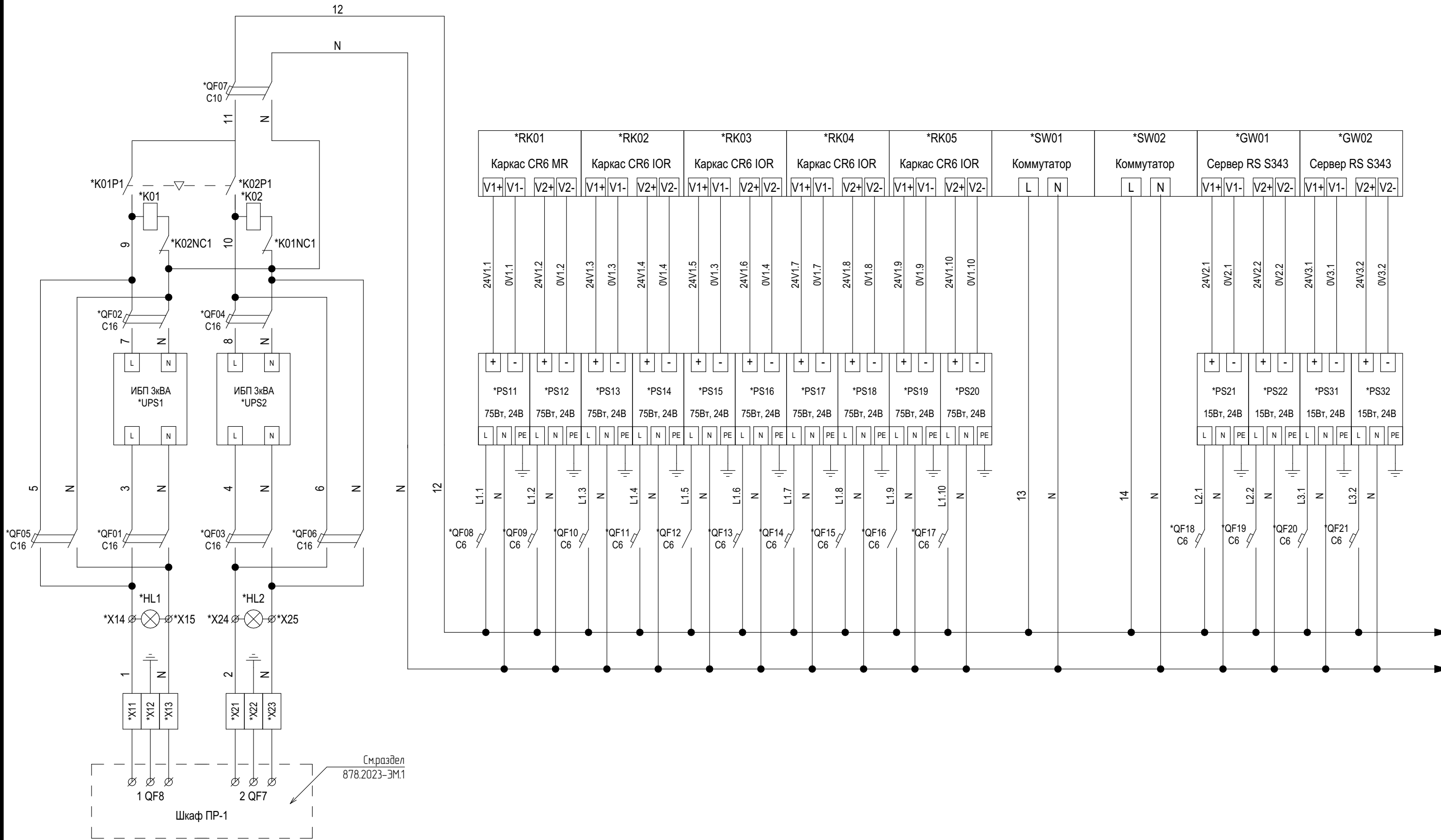
Принципиальная электрическая схема шкафа начало
